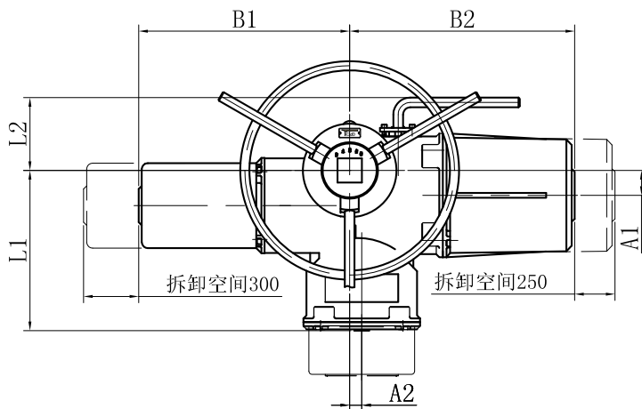
IMC25~60带BA外形尺寸
